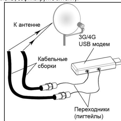
Схема 1 – пример подключения USB модема к МИМО облучателю параболической антенны
