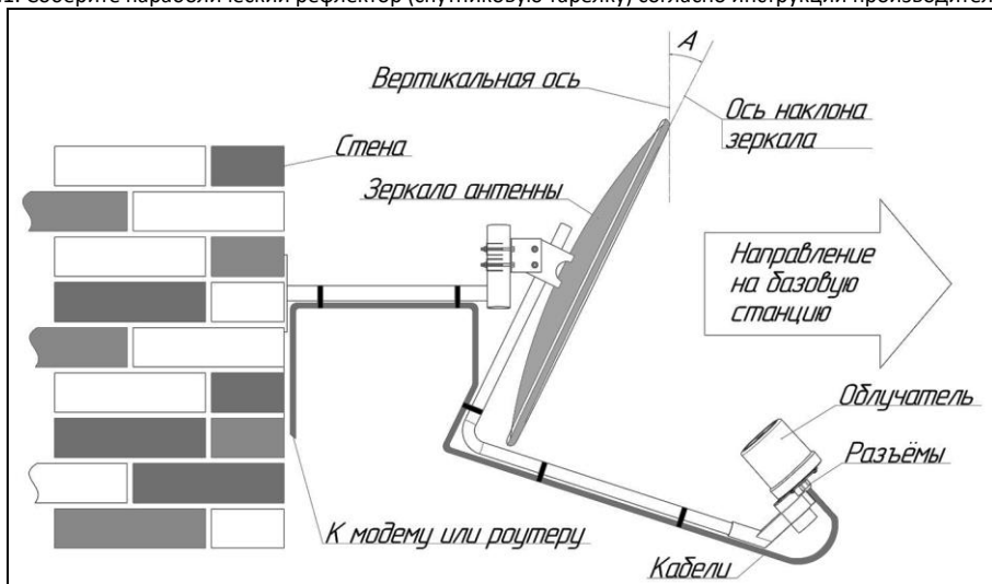
Рисунок 2 – Установка облучателя в держатель конвертера
