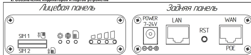
Рисунок 1 – Расположение индикаторов и портов SIM-инжектора
