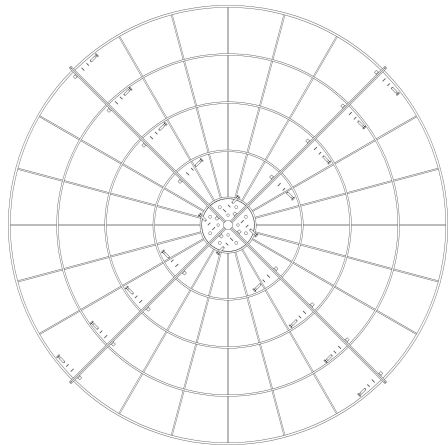
Шаг 2. Соберите параболический рефлектор из четырех составных частей.
