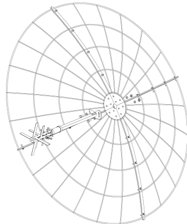
Шаг 3. Закрепите облучатель.
