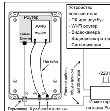
Пример размещения оборудования в гермобоксе
