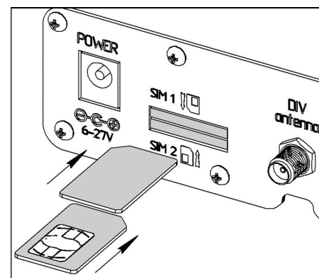
Рисунок 1- Установка SIM-карты
