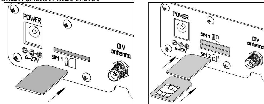
Рисунок 1 - Установка SIM-карт в роутеры KROKS Rt-Cse mQ-EC и KROKS Rt-Cse DS mQ-EC
