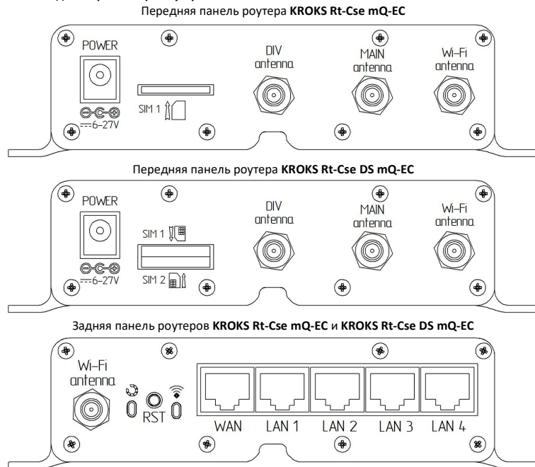
Схема 1 – Расположение индикаторов и портов устройства
