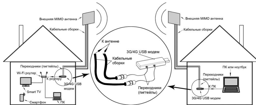
Схема 1 – пример подключения 4G WIMAX USB модема к MIMO антенне
