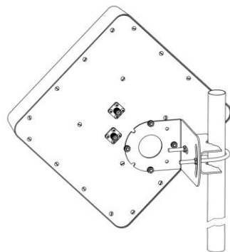
Рисунок 3 – X-поляризация
