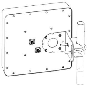
Рисунок 2 – монтаж антенны на мачте
