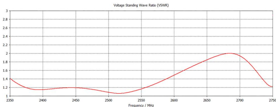
График КСВ в рабочем диапазоне частот
