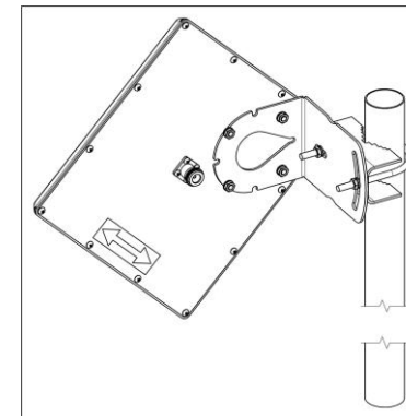
Рисунок 4 – X-поляризация
